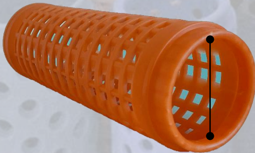
PUNTA DEL TUBO Ø I.P 57 mm
