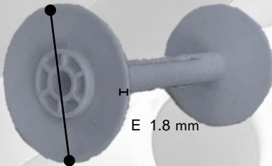
BASE DEL CARRETE Ø I.B 60 mm
