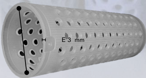
BASE DEL TUBO Ø I.B 54 mm
